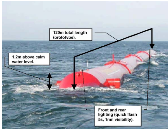
Fig. 4.5. OPD Pelamis WEC device.
